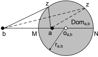
Fig. 16. Apollonius circle
